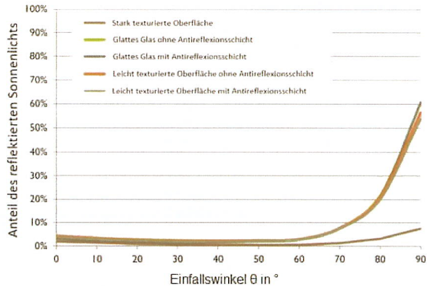
Abbildung 4: Anteil des reflektierten Sonnenlichts in Abhängigkeit zum Einfallswinkel, dargestellt für unterschiedliche Modulglastypeen - Quelle: [4], modifiziert
